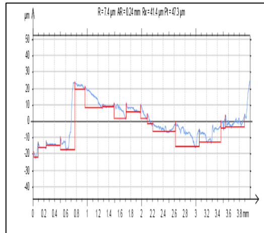
Fig 8: V=775.273m/min,F=32mm/min.,D=0.5mm
