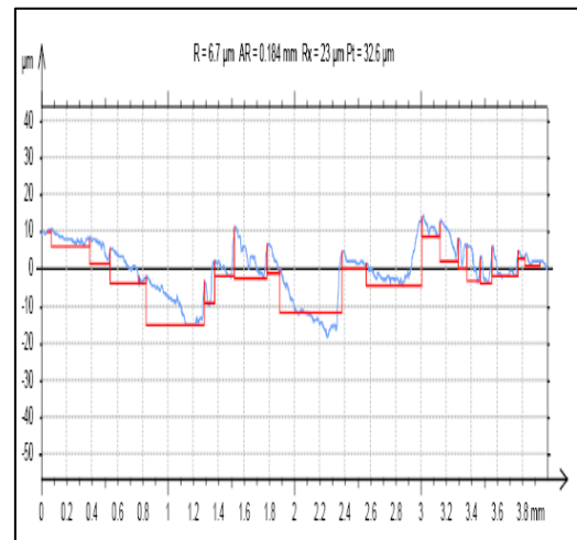
Fig 8: V=775.273m/min,F=32mm/min.,D=0.5mm
