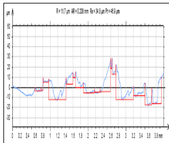
V=775.273m/min,F=32mm/min.,D=1.00mm
